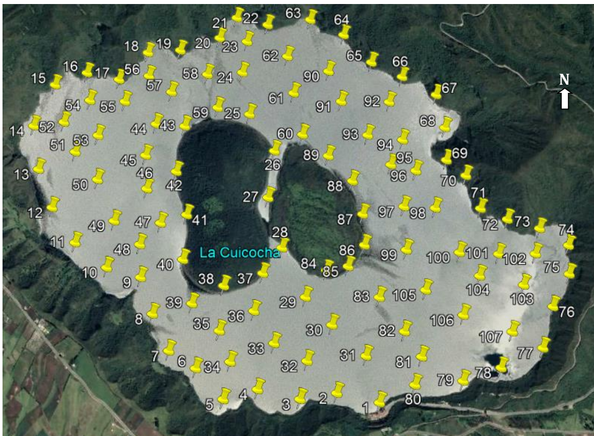
Figura 3. Esquema de la distribución de puntos de medición de CO 2 durante la campaña de Mayo 2019.
