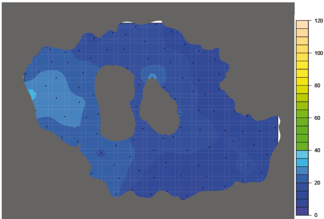
Figura 4. Distribución del flujo de CO 2 (g/m 2 /día) en la Laguna Cuicocha durante Mayo 2019.
