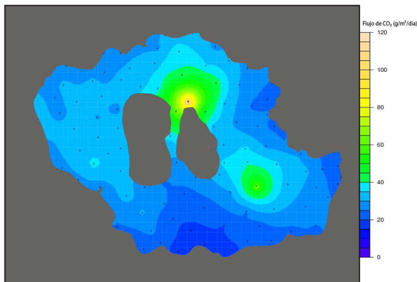
Figura 3. Distribución del flujo de CO 2 (g/m 2 /día) en la Laguna Cuicocha durante Enero 2019.
