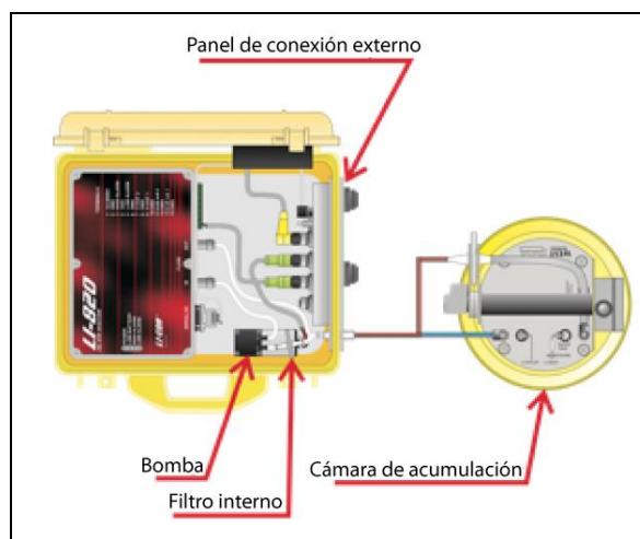
Figura 1. Configuración del instrumento de medición. Tomado del manual del usuario (WestSystems).
