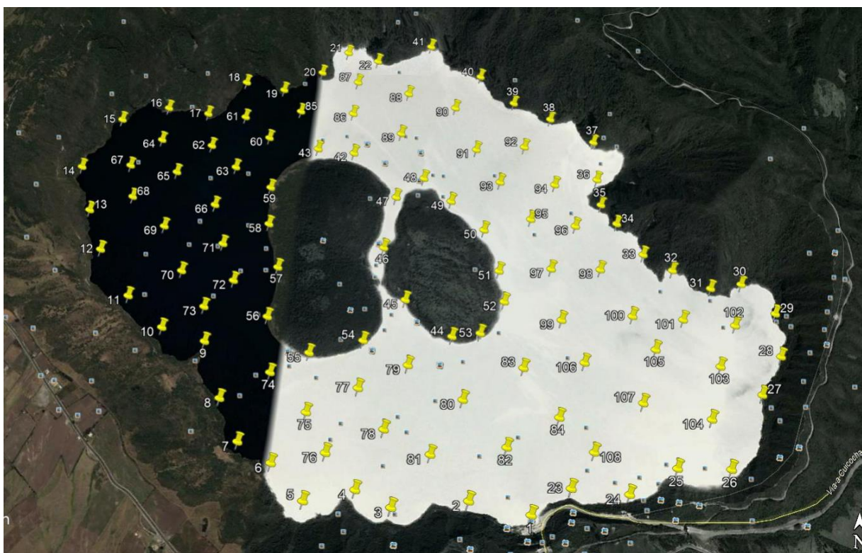
Figura 2. Esquema de la distribución de puntos de medición de CO 2 durante la campaña de Mayo 2018.
