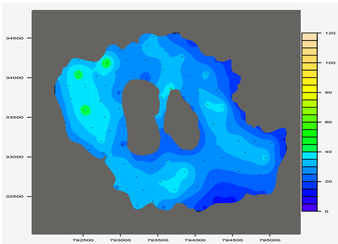
Figura 3. Distribución del flujo de CO 2 (g/m 2 /día) en la Laguna Cuicocha durante Mayo 2018.
