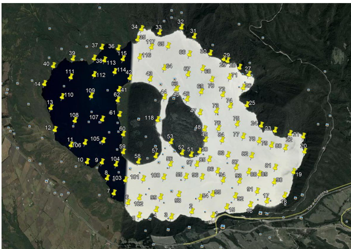
Figura 2. Esquema de la distribución de puntos de medición de CO 2 durante la campaña de Marzo 2018.
