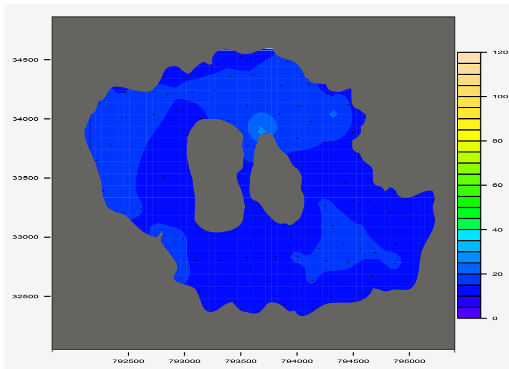
Figura 3. Distribución del flujo de CO 2 (g/m 2 /día) en la Laguna Cuicocha durante Marzo 2018.
