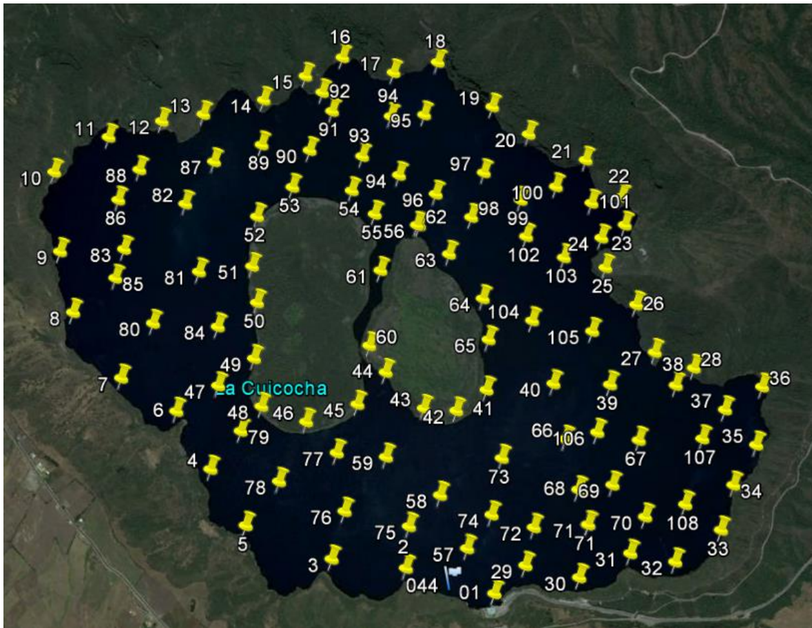
Figura 2. Esquema de la distribución de puntos de medición de CO 2 durante la campaña de Noviembre 2017.
