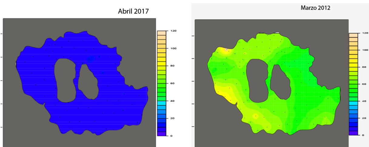
Figura 3. (a) Distribución del flujo de CO 2 (g/m 2 /día) en la Laguna Cuicocha durante Agosto 2017. (b) Gráficos comparativos de la mayor (Marzo 2012) y menor (Abril 2017) emisión de CO 2 registrada en esta laguna desde el año 2011. Todos los gráficos están representando utilizando una misma escala para la emisión de CO 2 .
