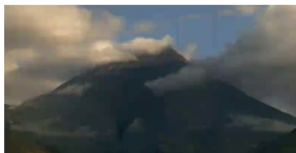
Foto: Cámara OVT. Volcán parcialmente despejado. 2019/10/15 16:50 TL
