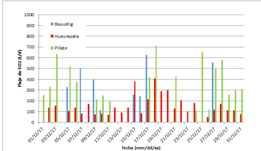
Figura 2. Representación del flujo diario de SO 2 , registrado por las estaciones Huayrapata, Bayushig y Pillate del volcán Tungurahua durante diciembre de 2017.
