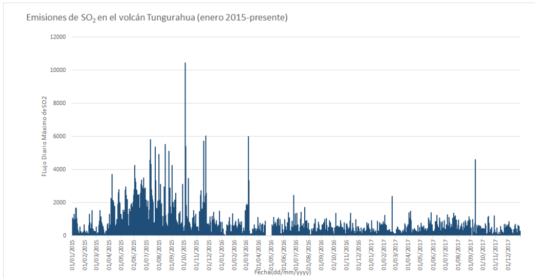
Figura 3. Gráfico del flujo diario máximo del SO 2 (t/d) registrado en el volcán Tungurahua entre enero 2015 y diciembre 2017.
