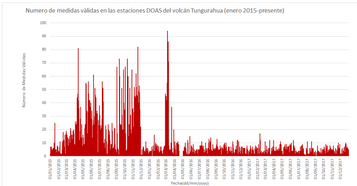
Figura 5.- Número de medidas válidas, registradas en el volcán Tungurahua entre enero 2015 y diciembre 2017.
