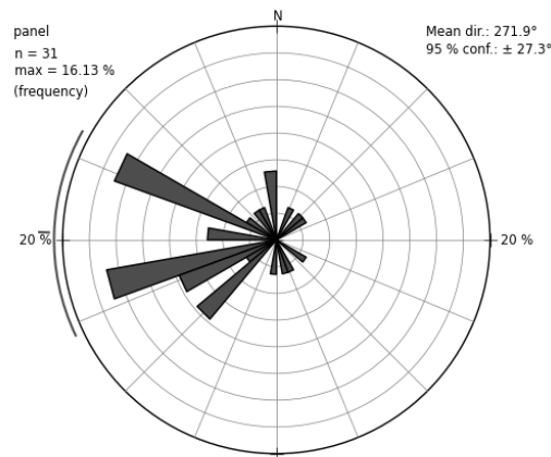
Figura 1.- Direcciones preferenciales del viento en el volcán Tungurahua para el mes de diciembre de 2017.
