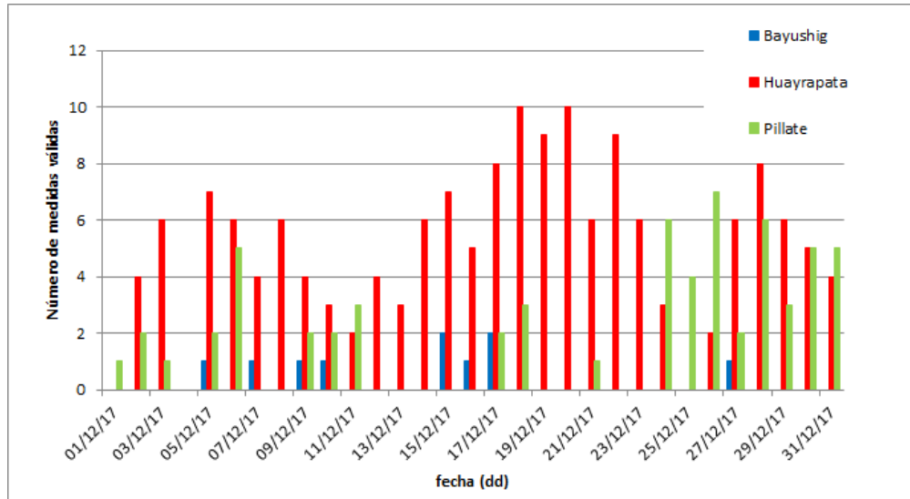
Figura 4. Representación del número de medidas válidas, registrado por las estaciones Huayrapata, Bayushig y Pillate del volcán Tungurahua durante diciembre de 2017.
