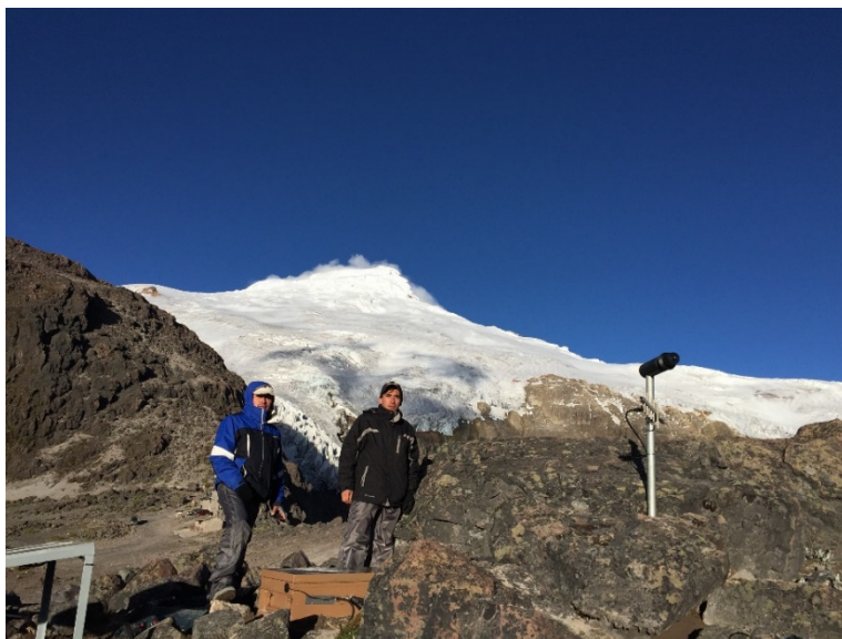
Fig 6: Instalación estación DOAS Cayambe Refugio
