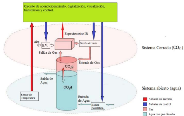
Fig: Medidor de CO2 terminado y esquema del funcionamiento
