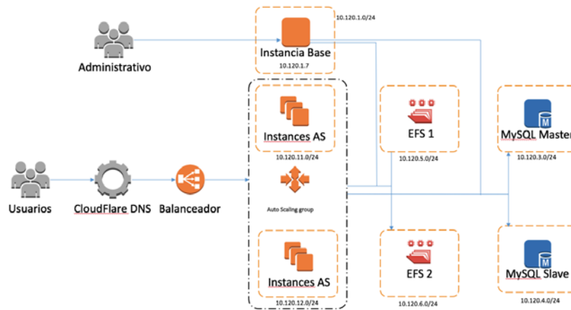
Figura 1. Esquema de la arquitectura para alta disponibilidad de la página web
