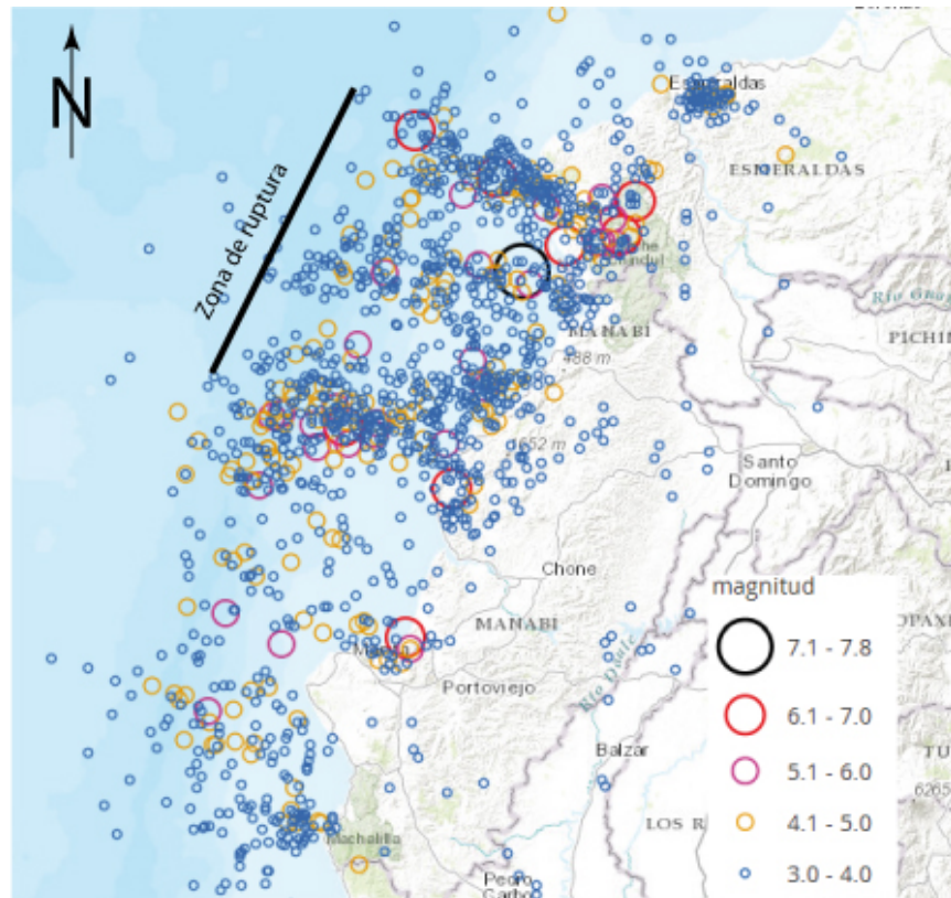
Figura 2. Distribución de la sismicidad luego de la ocurrencia del sismo de Pedernales del 16 de abril de 2016. El sismo ocurrió a lo largo del plano de falla o interface de contacto entre la placa continental superior y la placa oceánica que se subduce, con un mecanismo inverso. La zona de ruptura principal se encuentra entre el sur de punta Galera hasta Cabo Pasado con un largo de 140 km aproximadamente y cerca de 100 km de ancho, tal como muestra la distribución de réplicas (Figuras 1 y 2).
