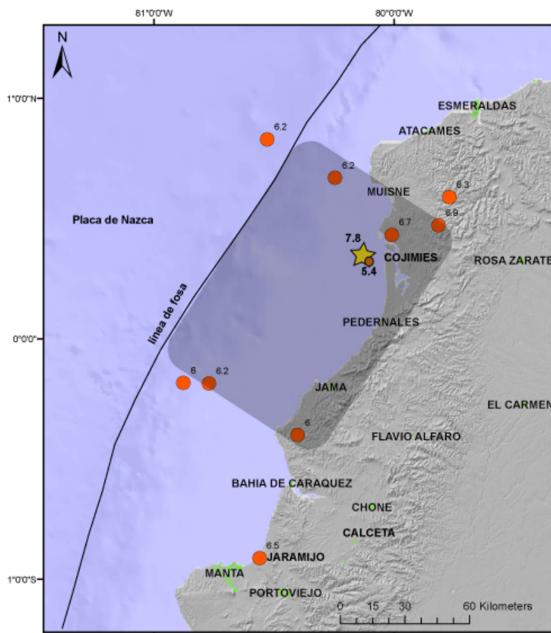
Figura 1. Localización del sismo de Pedernales (estrella amarilla), su premonitor (círculo naranja pequeño) y de las principales réplicas (círculos rojos). La zona sombreada corresponde aproximadamente al área de
